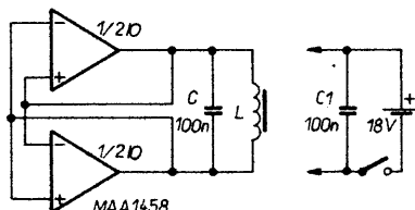
Obr. 1. Schéma vysílače
